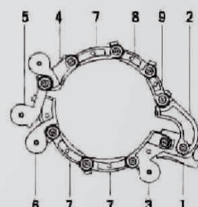
Fig I, 25.1/2"-27"
